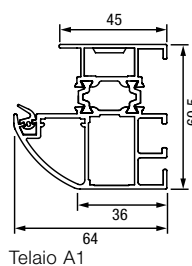
Telaio A1
