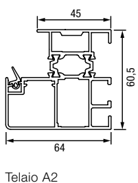
Telaio A2
