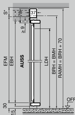
Sezione verticale portone senza battuta inferiore
