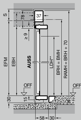
Sezione verticale portone con battuta inferiore
