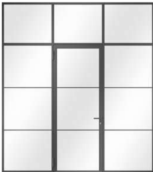
1-flüglige Drehflügeltür mit Seitenteilen und Oberlichtern sowie 2 horizontalen Sprossen, Glashalteleiste Slim
