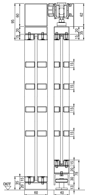
Vertikalschnitt 2-flüglige Stahl-Lofttür mit Seitenteil
