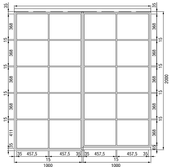
2-flüglige Stahl-Lofttür mit Seitenteil
