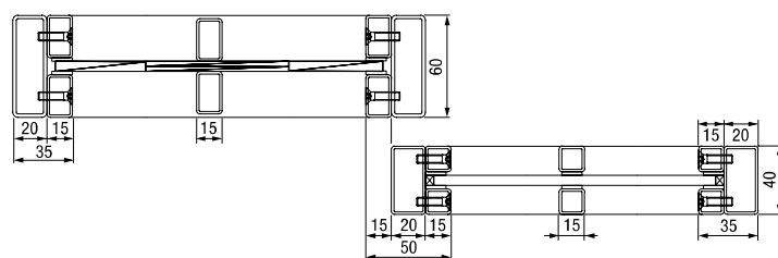
Horizontalschnitt 2-flüglige Stahl-Lofttür mit Seitenteil
