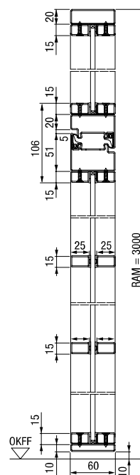
Vertikalschnitt 1-flügelige Stahl-Lofttür mit Oberlicht
